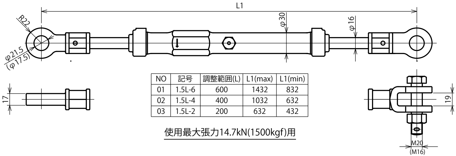
ワイヤターンバックル A形
